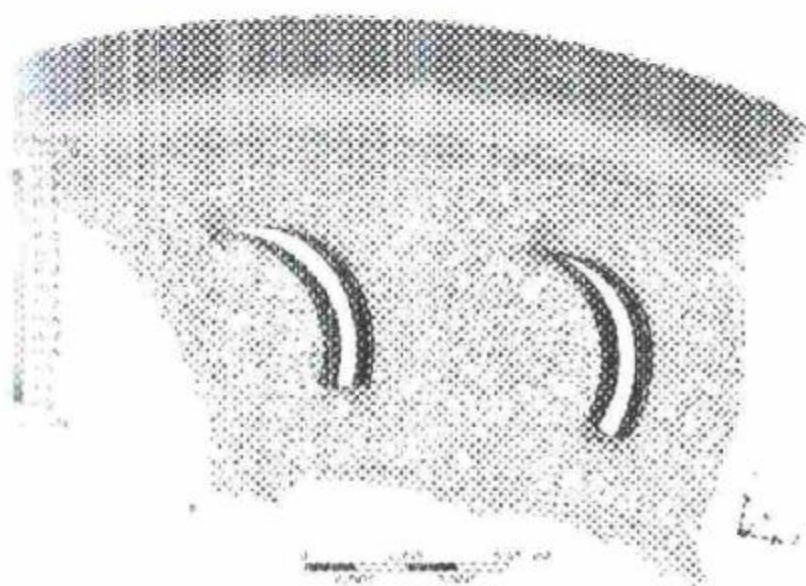
Рис. 3. Картина течії у міжлопатевих каналах доцентрового ступеню варіанту 1
